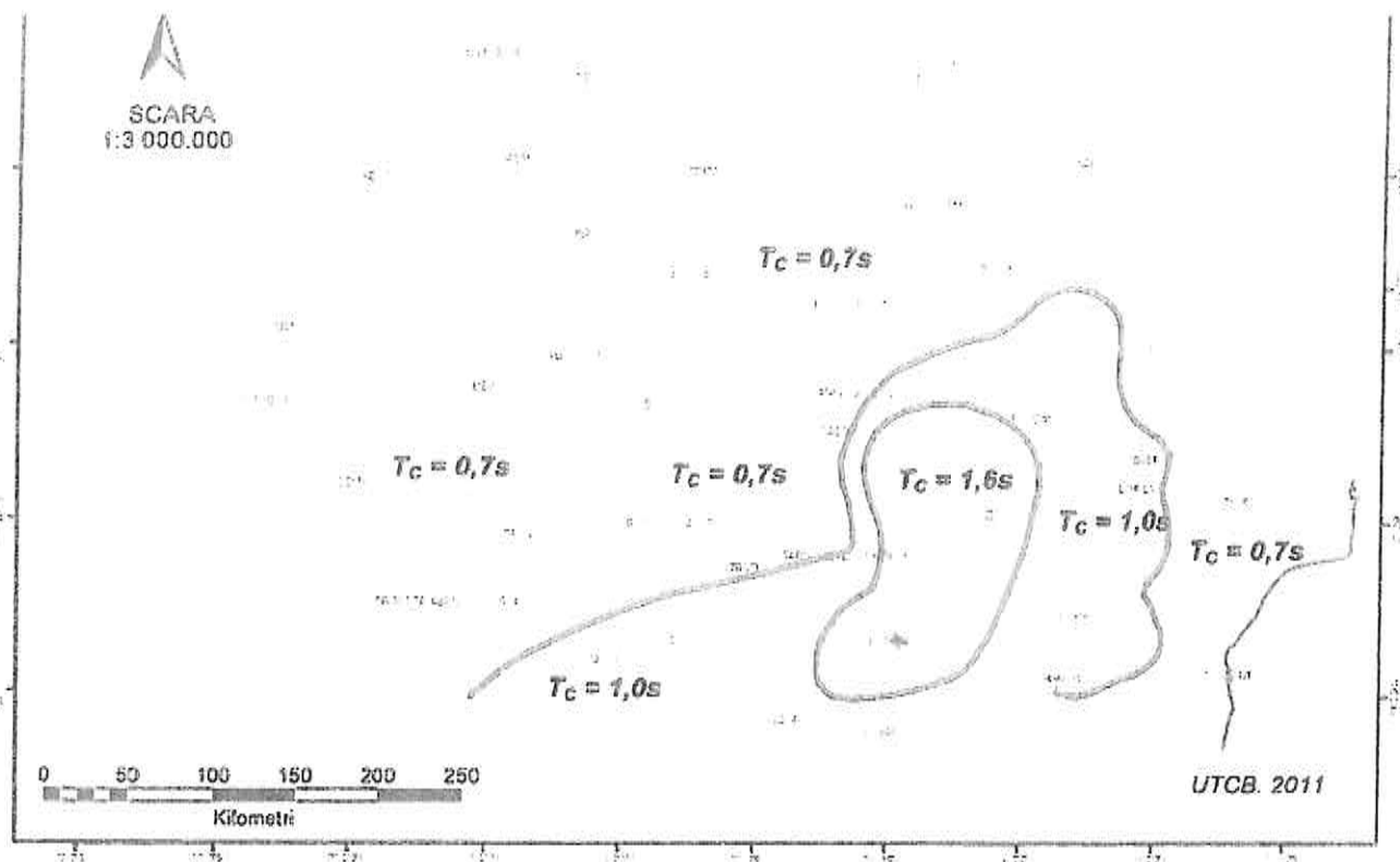
Zonarea teritoriului României în termeni de perioada de control (colt), T_c a spectrului de răspuns
